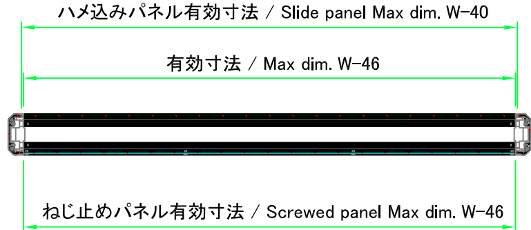
A-A ( 1 : 8 )
