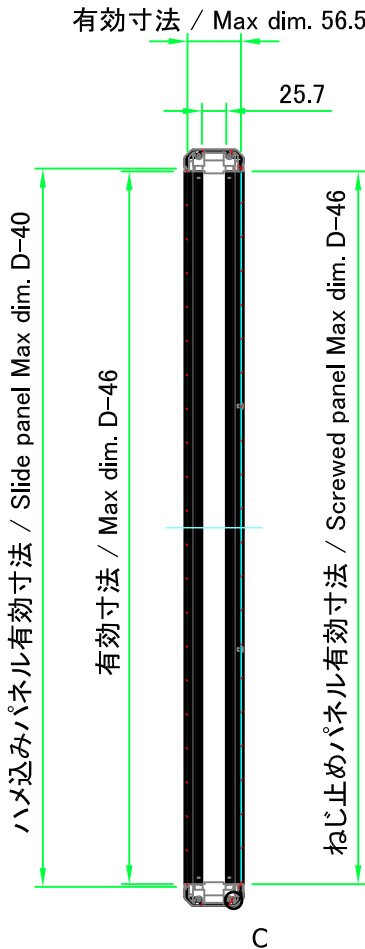
B-B ( 1 : 8 )
